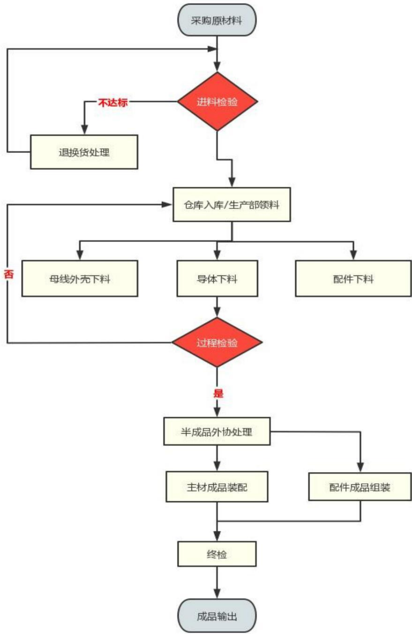
图 3.2 工艺流程图
